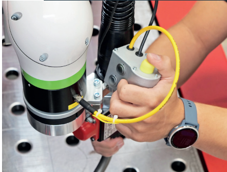
Programación sencilla de la trayectoria de soldadura mediante guiado directo de la antorcha
